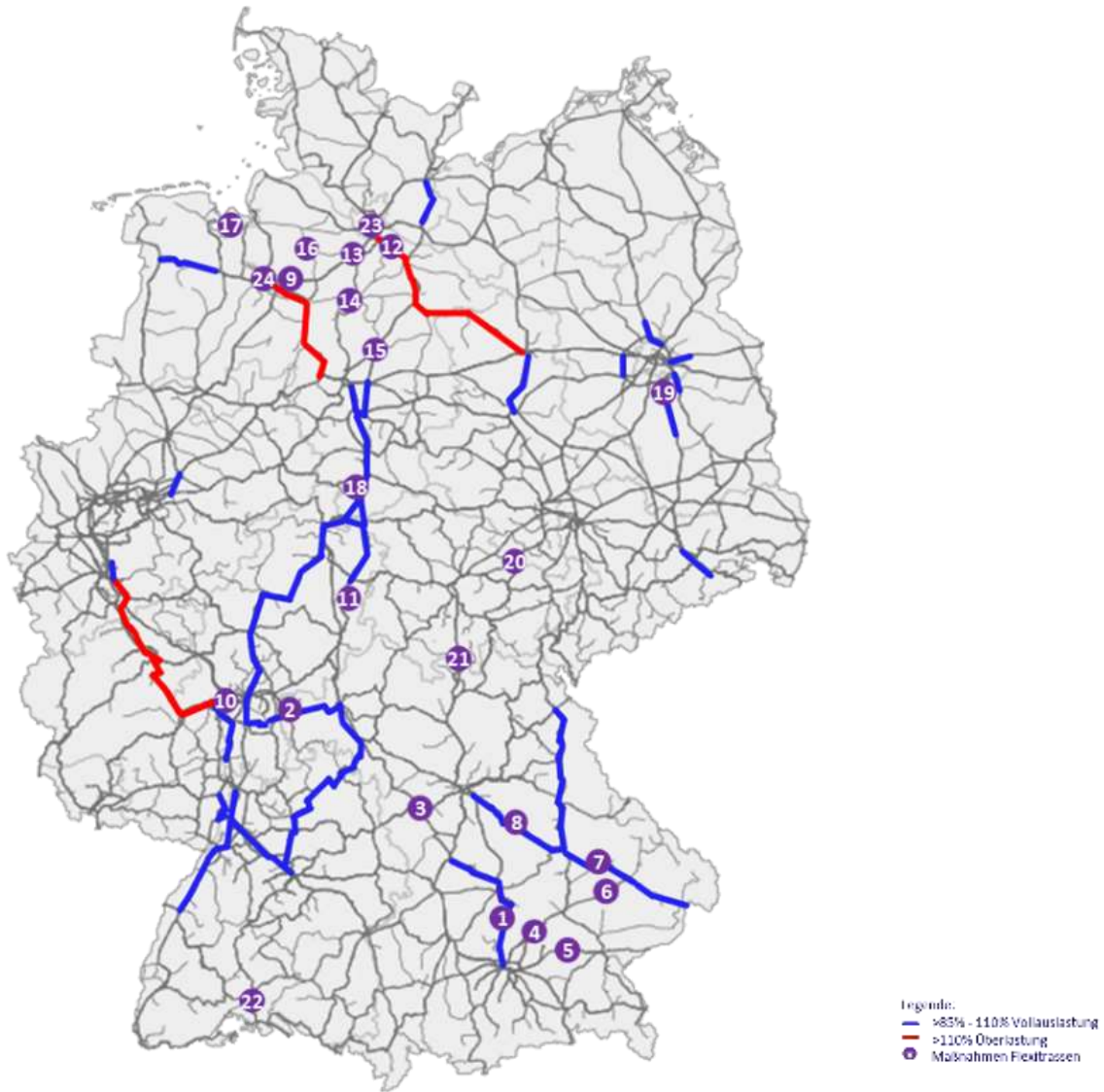
Abb. 1: Flexitrassen-Maßnahmen
